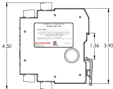
SST7000 / SST7100
